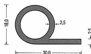
Artikel-Nr. 540.5188 EPDM · 68° ShoreA · schwarz VE: Bund á 25m
