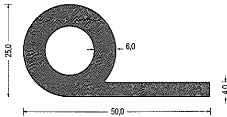
Artikel-Nr. 540.5252 EPDM · 60° ShoreA · schwarz VE: Bund á 25m
