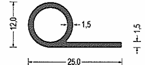
Artikel-Nr. 540.5122 EPDM · 60° ShoreA · schwarz VE: Bund á 50m
