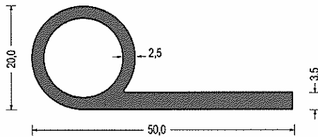
Artikel-Nr. 540.5206 EPDM · 60° ShoreA · schwarz VE: Bund á 25m
