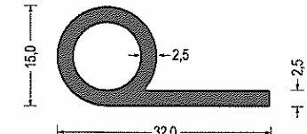
Artikel-Nr. 540.5154 EPDM · 65° ShoreA · schwarz VE: Bund á 50m
