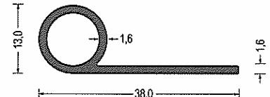
Artikel-Nr. 540.5133 EPDM · 70° ShoreA · schwarz VE: Bund á 50m
