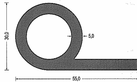
Artikel-Nr. 540.5301 EPDM · 65° ShoreA · schwarz VE: Bund á 25m
