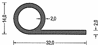
Artikel-Nr. 540.5141 EPDM · 65° ShoreA · schwarz VE: Bund á 50m
