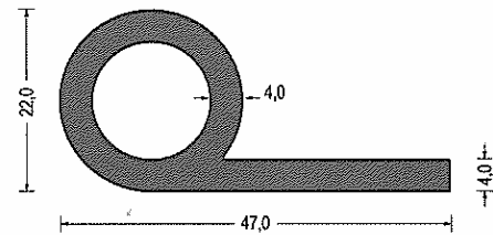
Artikel-Nr. 540.5224 EPDM · 70° ShoreA · schwarz VE: Bund á 25m
