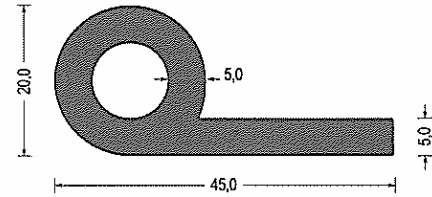
Artikel-Nr. 541.5201 CR · 45° ShoreA · schwarz VE: Bund á 25m
