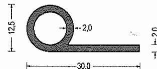
Artikel-Nr. 540.5127 EPDM · 70° ShoreA · schwarz VE: Bund á 50m
