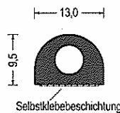
Artikel-Nr. 588.6202 EPDM · schwarz · SK mit Hohlkammer VE: Spule á 100m als Montagehilfe einseitig selbstklebend
