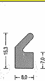
Artikel-Nr. 580.7110 EPDM · grau VE: Bund á 50m
