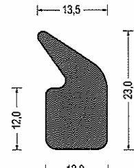
Artikel-Nr. 581.5542 CR · schwarz VE: Bund á 50m
