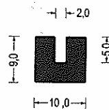
Artikel-Nr. 580.7361 EPDM - schwarz VE: Bund á 50m
