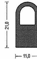
Artikel-Nr. 580.6882 EPDM · schwarz mit Hohlkammer VE: Bund á 50m
