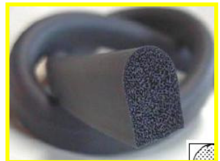
Artikel-Nr. 580.6121 EPDM · grau VE: Bund á 50m
