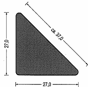
Artikel-Nr. 580.5472 EPDM · schwarz VE: Bund á 25m
