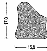
Artikel-Nr. 580.6971 EPDM · grau VE: Bund á 50m
