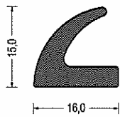
Artikel-Nr. 580.6172 EPDM · schwarz VE: Bund á 25m
