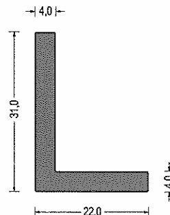
Artikel-Nr. 580.6512 EPDM · schwarz VE: Bund á 25m
