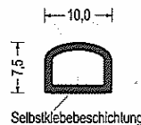
Artikel-Nr. 588.6672 EPDM · schwarz · SK mit Hohlkammer VE: Spule á 150m als Montagehilfe einseitig selbstklebend
