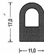
Artikel-Nr. 580.8882 EPDM · schwarz mit Hohlkammer VE: Bund á 50m
