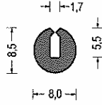
Artikel-Nr. 580.6412 EPDM · schwarz VE: Bund á 200m
