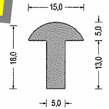
Artikel-Nr. 580.7041 EPDM · grau VE: Bund á 50m
