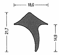
Artikel-Nr. 580.6022 EPDM · schwarz VE: Bund á 50m
