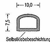
Artikel-Nr. 588.6676 EPDM · grau · SK mit Hohlkammer VE: Spule á 150m als Montagehilfe einseitig selbstklebend
