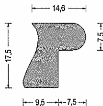
Artikel-Nr. 580.5211 EPDM · grau VE: Bund á 50m
