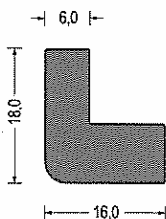
Artikel-Nr. 580.7442 EPDM · schwarz VE: Bund á 50m
