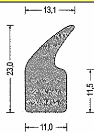
Artikel-Nr. 580.7321 EPDM · grau VE: Bund á 50m
