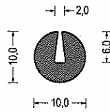
Artikel-Nr. 580.5022 EPDM · schwarz VE: Bund á 50m
