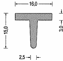
Artikel-Nr. 580.7781 EPDM · grau VE: Bund á 25m
