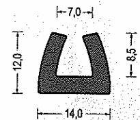
Artikel-Nr. 580.7077 EPDM - schwarz VE: Bund á 50m
