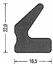
Artikel-Nr. 580.7872 EPDM · schwarz VE: Bund á 25m
