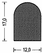
Artikel-Nr. 580.5618 EPDM · schwarz VE: Bund á 50m
