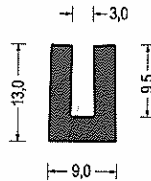
Artikel-Nr. 580.5962 EPDM - schwarz VE: Bund á 50m
