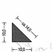
Artikel-Nr. 580.2172 EPDM · schwarz VE: Bund á 50m
