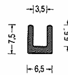
Artikel-Nr. 580.6935 EPDM - schwarz VE: Bund á 100m
