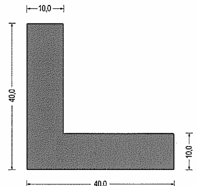
Artikel-Nr. 580.6632 EPDM · schwarz VE: Bund á 25m
