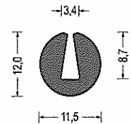
Artikel-Nr. 580.5332 EPDM · schwarz VE: Bund á 50m
