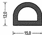
Artikel-Nr. 580.6772 EPDM · schwarz mit Hohlkammer VE: Bund á 100m
