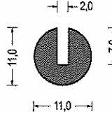
Artikel-Nr. 580.5357 EPDM · schwarz VE: Bund á 50m
