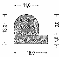
Artikel-Nr. 580.6611 EPDM · grau VE: Bund á 50m
