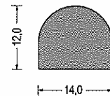
Artikel-Nr. 580.6121 EPDM · grau VE: Bund á 50m
