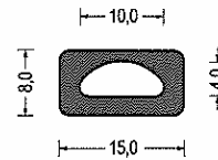
Artikel-Nr. 580.4472 EPDM · schwarz VE: Bund á 100m
