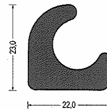
Artikel-Nr. 580.8703 EPDM · schwarz VE: Bund á 25m
