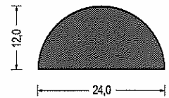
Artikel-Nr. 580.5972 EPDM · schwarz VE: Bund á 50m
