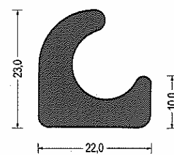
Artikel-Nr. 580.8703 EPDM · schwarz VE: Bund á 25m
