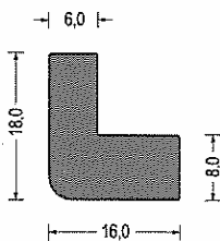
Artikel-Nr. 580.7442 EPDM · schwarz VE: Bund á 50m
