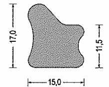
Artikel-Nr. 580.7071 EPDM · grau VE: Bund á 50m
