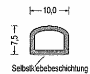
Artikel-Nr. 588.6676 EPDM · grau · SK mit Hohlkammer VE: Spule á 150m als Montagehilfe einseitig selbstklebend
