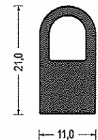
Artikel-Nr. 580.6882 EPDM · schwarz mit Hohlkammer VE: Bund á 50m
