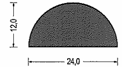
Artikel-Nr. 580.5972 EPDM · schwarz VE: Bund á 50m
