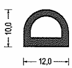
Artikel-Nr. 580.7788 EPDM · schwarz mit Hohlkammer VE: Bund á 100m
